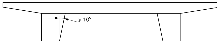
Figuur 45: Dwarsdoorsnede brug met afgeschuivde hoofdliggers
