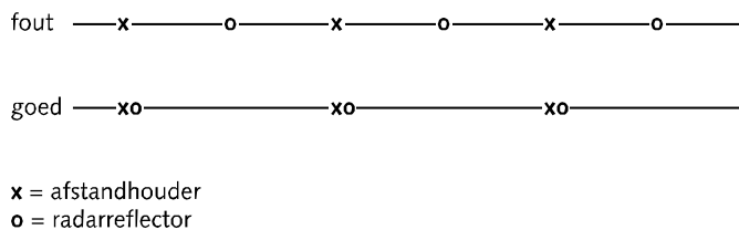
Figuur 18: Plaats afstandhouders hoogspanningsleidingen
