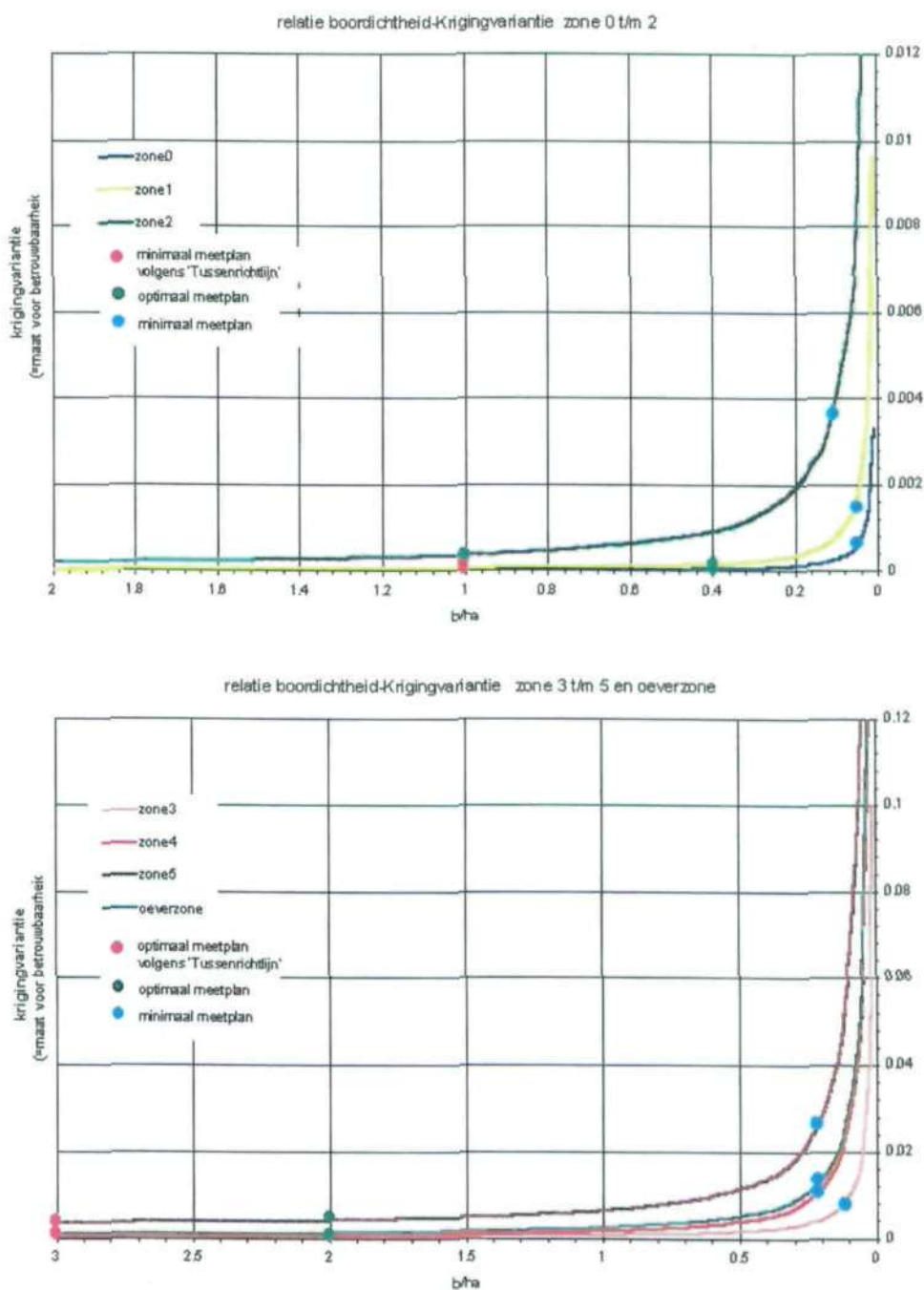
Figuur B2.1: Krigingvarianties voor de verschillende meetpunt-dichtheden
