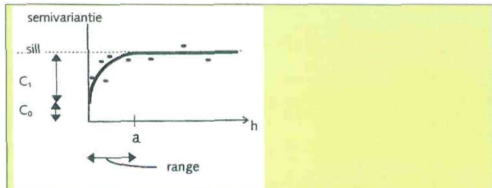
Voorbeeld van een semivariogram ter verklaring van tabel B1.3 (Kruyt en Hazelhoff, 2000)
