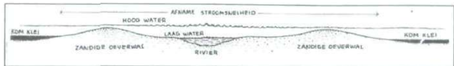
Figuur 2.3: Dwarsprofiel door een onbeteugelde rivier (RWS-RIZA, 1998)
