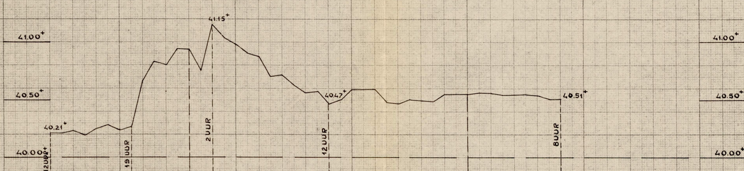
PEILSCHAAL BEN STUW BORGHAREN K.M. RAAI 15.590 OORWAARNEMINGEN VAN 13 OCT. 12 UUR TOT 15 OCT. 8 UUR
