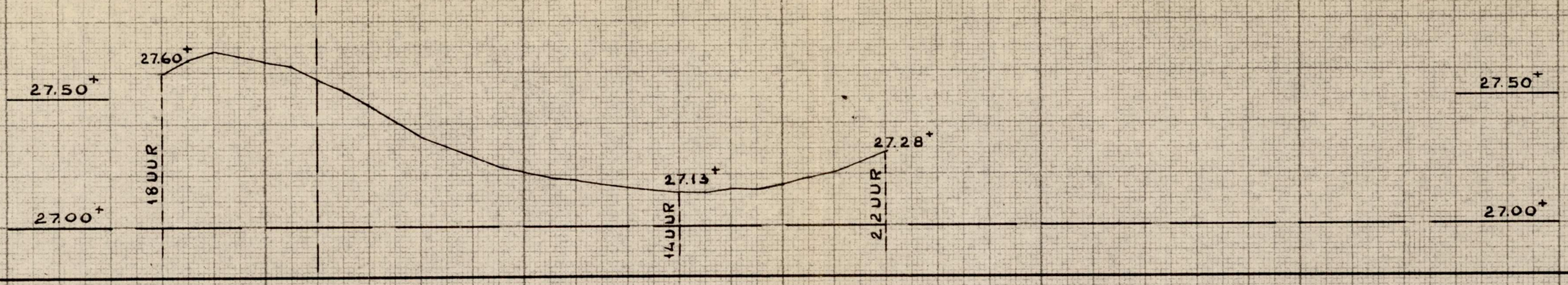
PEILSCHAAL GREVENBICHT K.M. RAAI 44.945 OORWAARNEMINGEN VAN 15 OCT. 18 UUR TOT 16 OCT. 22 UUR
