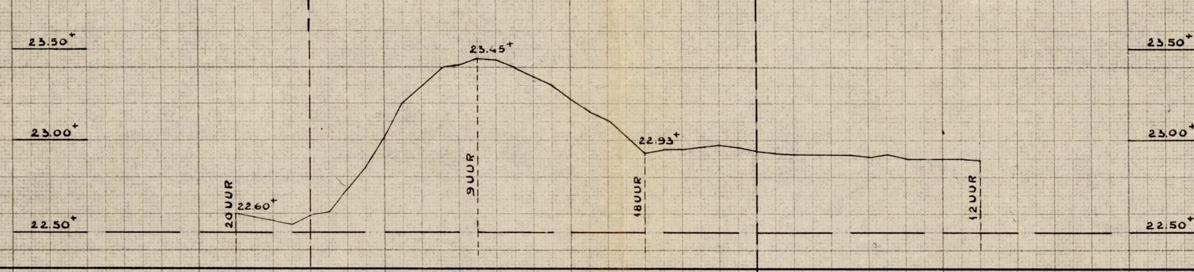
PEILSCHAAL MAASBRACHT K.M. RAAI 65.500 OORWAARNEMINGEN VAN 13 OCT. 20 UUR TOT 15 OCT. 12 UUR
