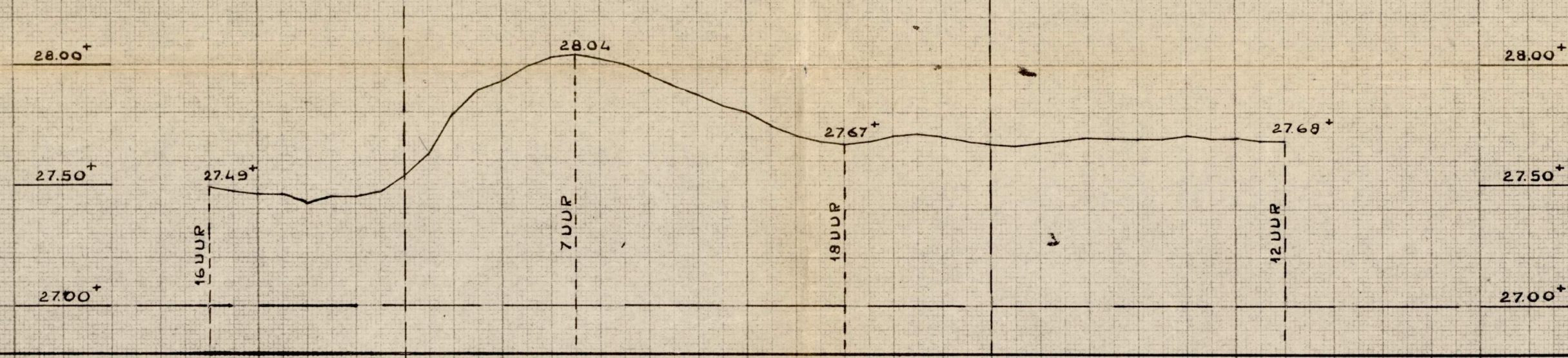
PEILSCHAAL MAESEYCK K.M. RAAI 52.450 OORWAARNEMINGEN VAN 15 OCT. 20 UUR TOT 15 OCT. 12 UUR
