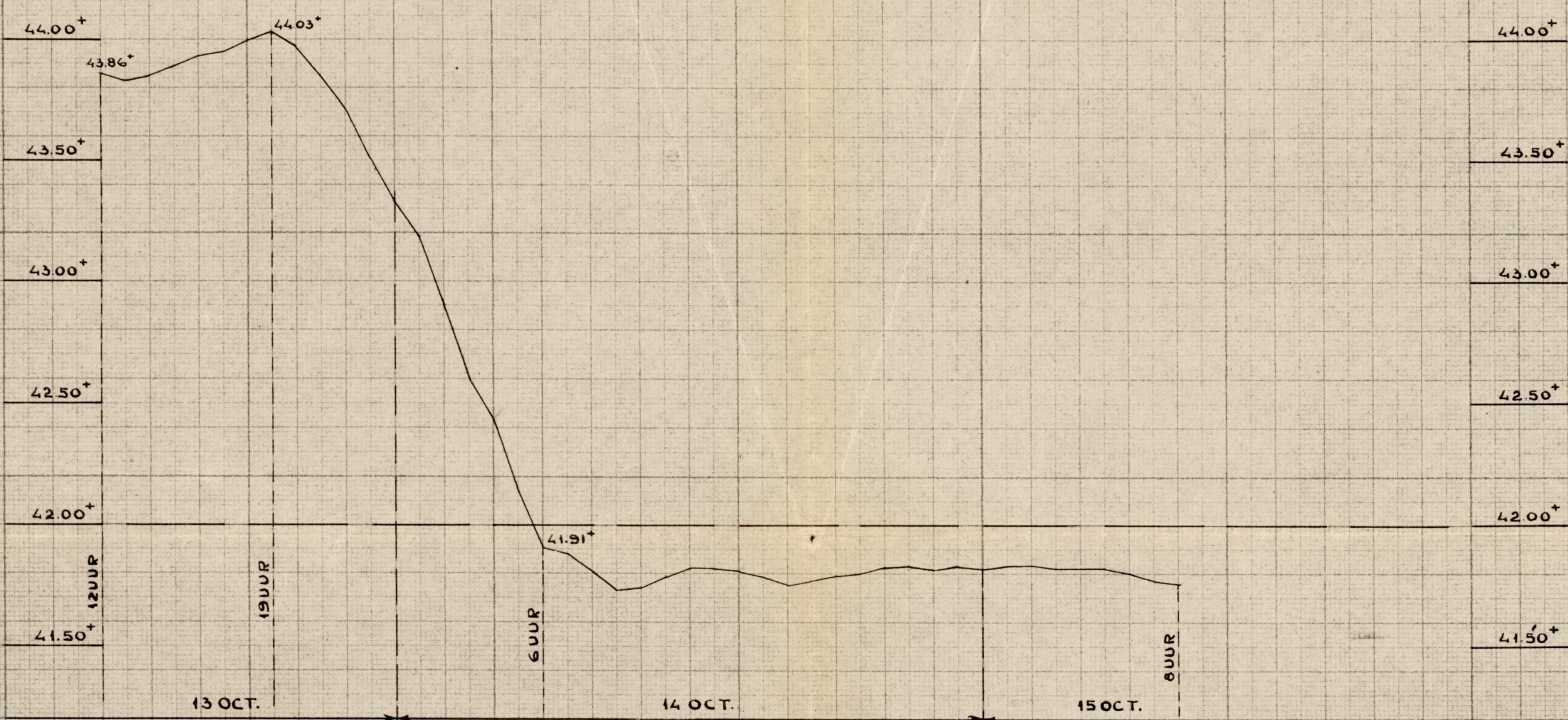
PEILSCHAAL BOVEN STUW BORGHAREN OORWAARNEMINGEN VAN 13 OCT. 12 UUR TOT 15 OCT. 8 UUR
