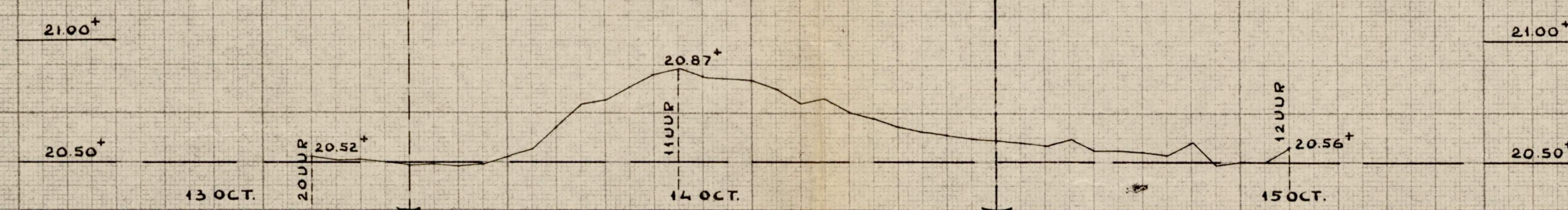
PEILSCHAAL MAASBRACHT K.M. RAAI 65.500 OORWAARNEMINGEN VAN 13 OCT. 20 UUR TOT 15 OCT. 12 UUR
