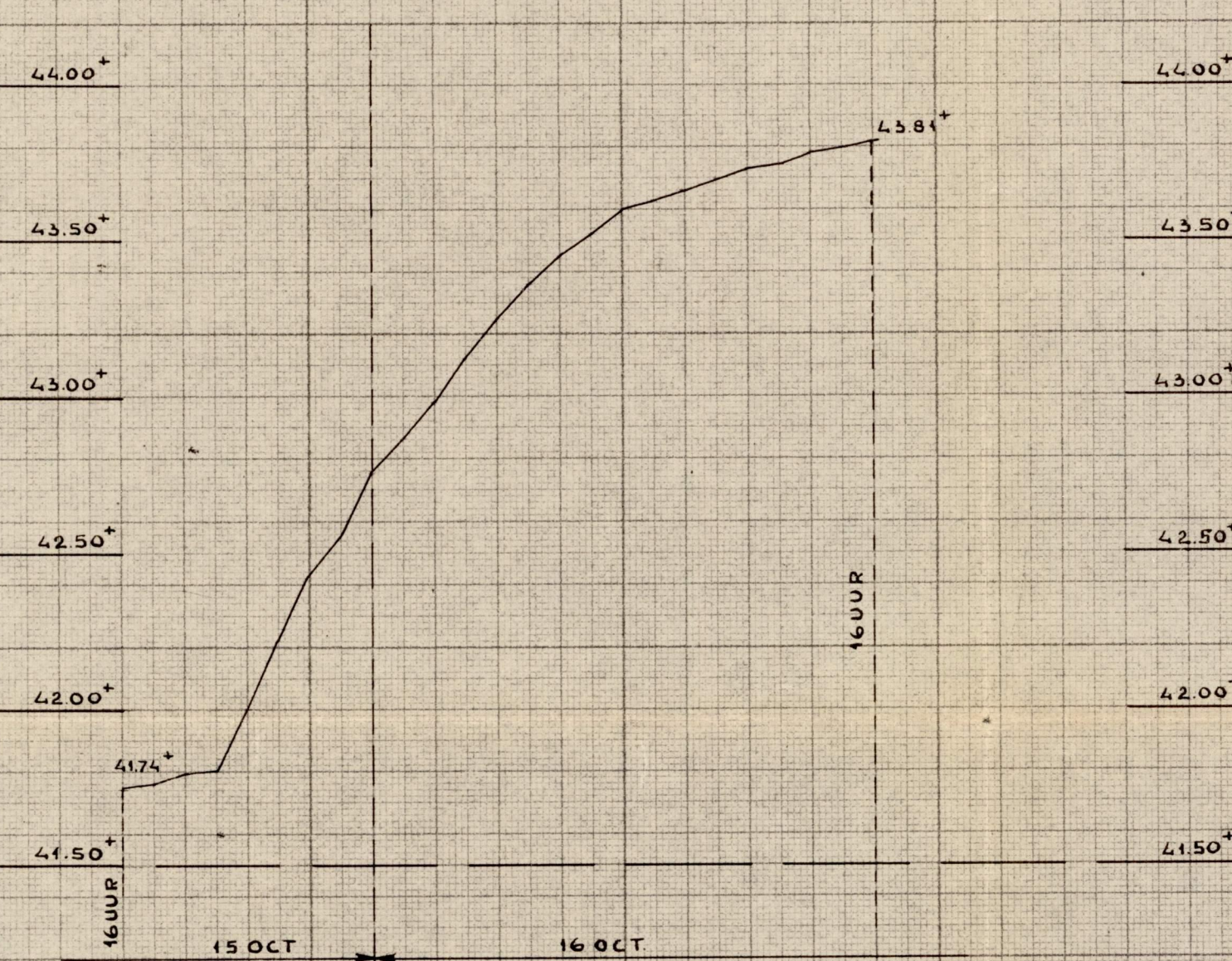
PEILSCHAAL BOVEN STUW BORGHAREN OORWAARNEMINGEN VAN 15 OCT. 16 UUR TOT 16 OCT. 16 UUR
