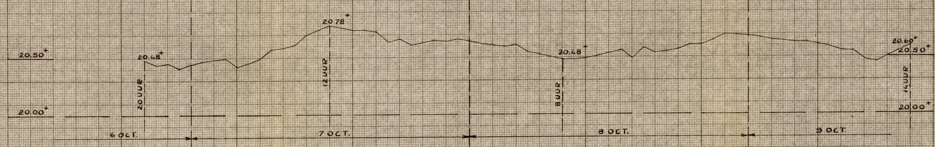
PEILSCHAAL MAASBRACHT K.M. RAAI 65.500 OORWAARNEMINGEN VAN 6 OCT. 20 UUR TOT 9 OCT. 14 UUR
