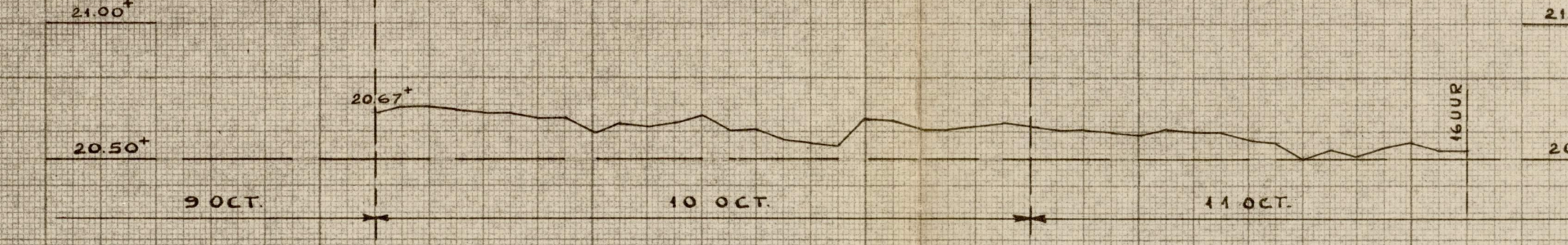
PEILSCHAAL MAASBRACHT K.M. RAAI 65.500 OORWAARNEMINGEN VAN 10 OCT. 0 UUR TOT 11 OCT. 16 UUR
