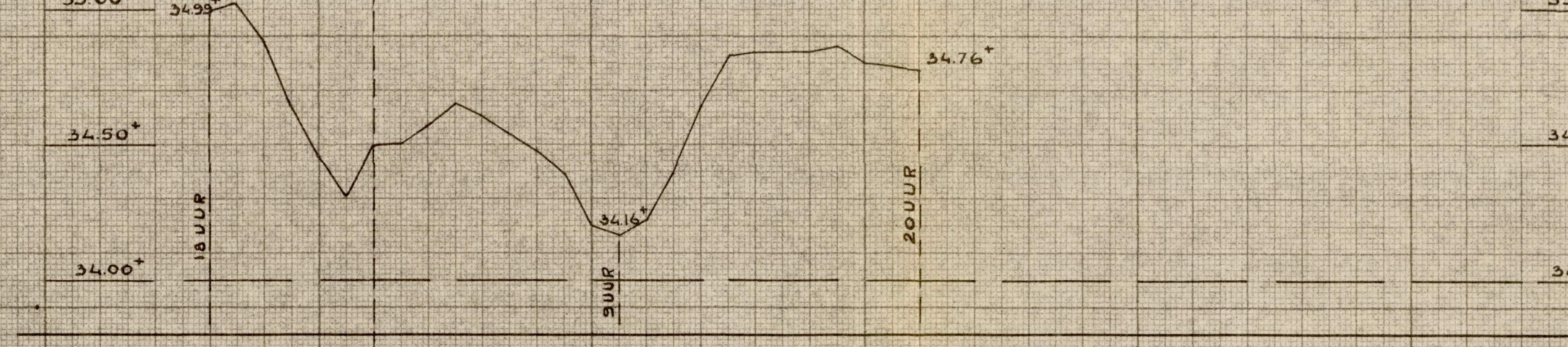
PEILSCHAAL ELSLOO K.M. RAAI 29.405 OORWAARNEMINGEN VAN 9 OCT. 18 UUR TOT 10 OCT. 20 UUR
