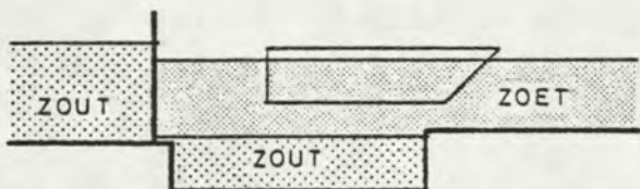
FASE ④ UIT-EN INVAREN SCHEPEN (VOLKERAK)
