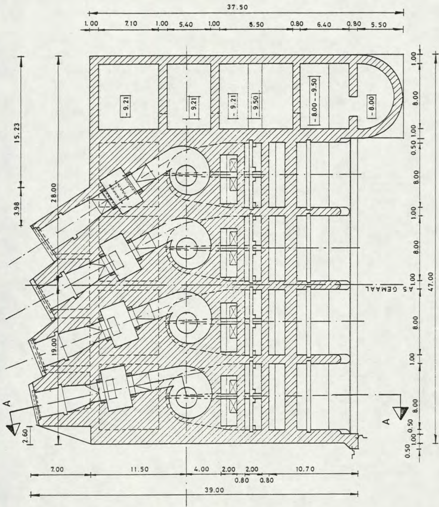
HORIZONTALE DOORSNEDE B-B GEMAAL
