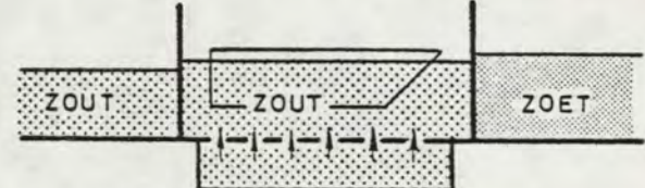
FASE ② OPWAARTS NIVELLEREN
