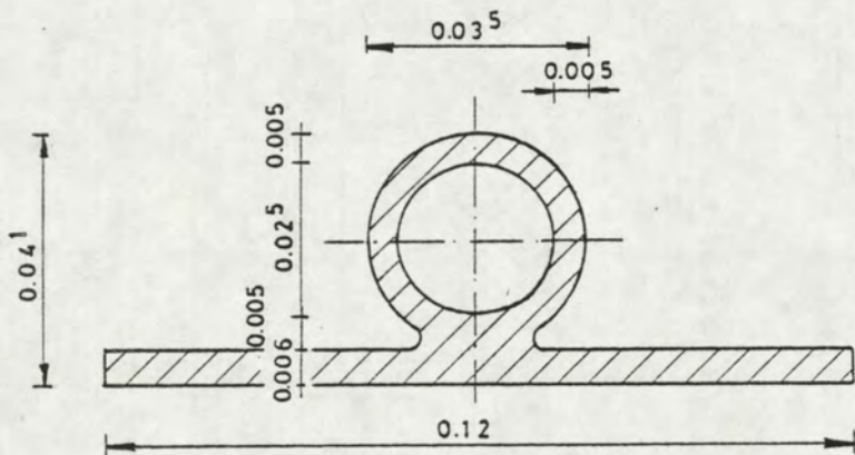
DETAIL RUBBER AFDICHTINGSPROFIEL
