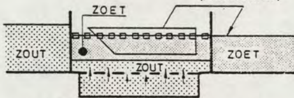
FASE ⑤ OPWAARTS UITWISSELEN
