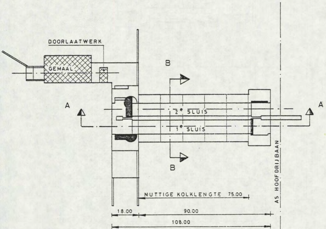
BOVENAANZICHT
