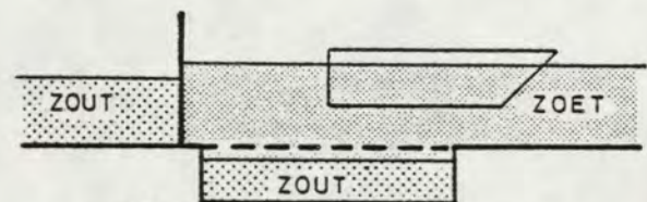
FASE ④ UIT-EN INVAREN SCHEPEN (VOLKERAK)
