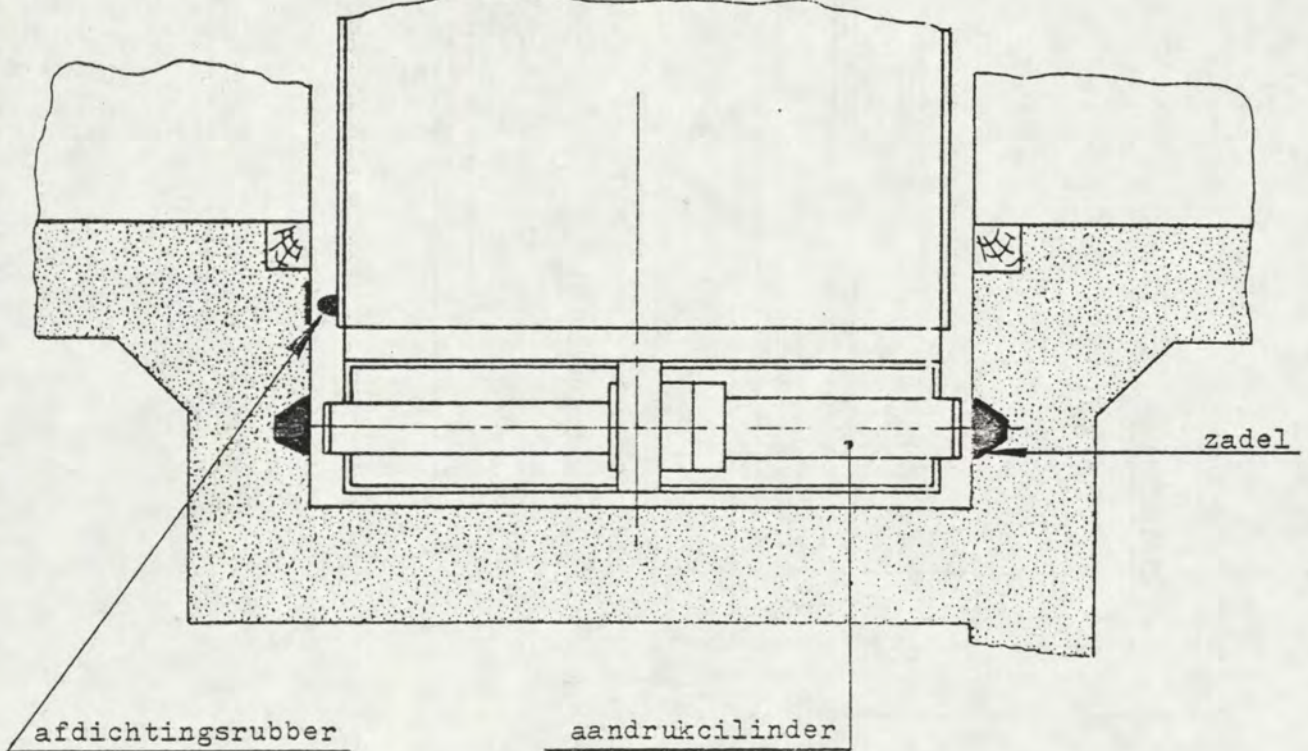
DEUR IN MIDDENSTAND
