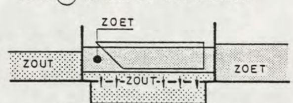
FASE ⑥ NEERWAARTS NIVELLEREN
