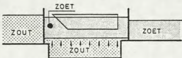
FASE ⑤ OPWAARTS NIVELLEREN
