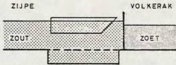
FASE ① INVAREN SCHEPEN (ZIJPE)
