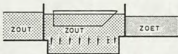
FASE ② NEERWAARTS NIVELLEREN
