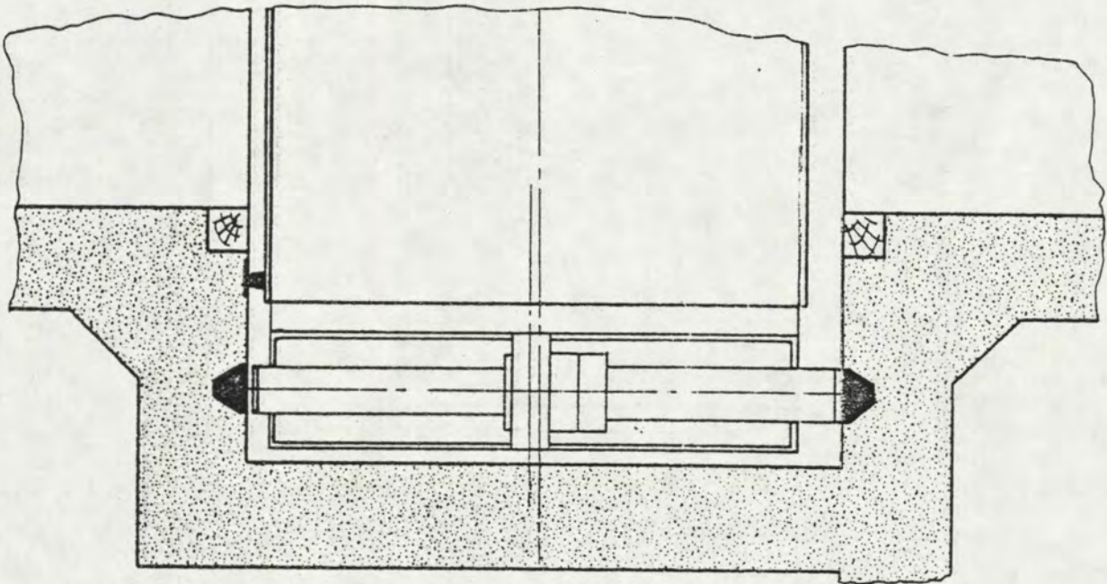
DEUR IN MIDDENSTAND
