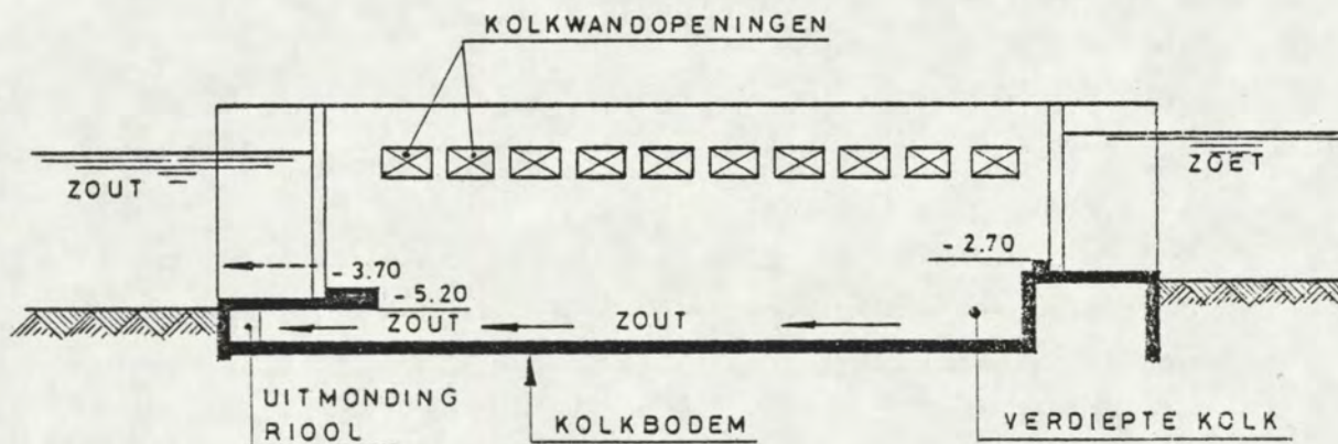
SCHEMATISCHE LENGTEDOORSNEDE
