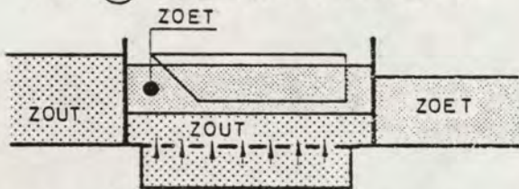
FASE ⑥ OPWAARTS NIVELLEREN
